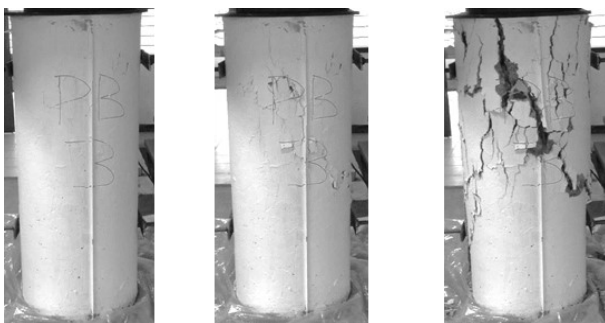
Gambar 9. Pola retak benda uji kolom lingkaran tulangan pengekuat tidak standar dengan perkuatan pen-binder
