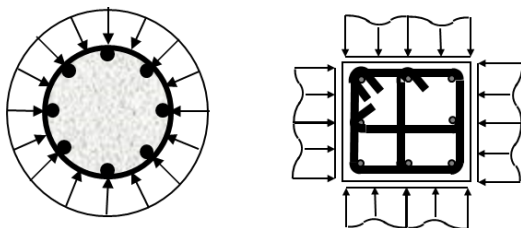
Gambar 3. Efektifitas aksi kekangan lateral pada pengekat spiral dan persegi
