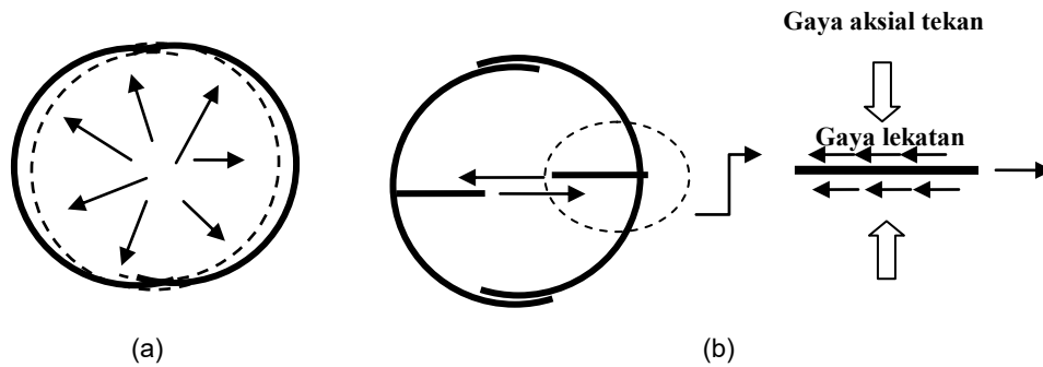
Gambar 4. Ilustrasi konsep pen-binder sebagai elemen pengikat (a) Pengekan lingkaran tanpa pen-binder (b) Pengekan lingkaran yang diberi pen-binder
