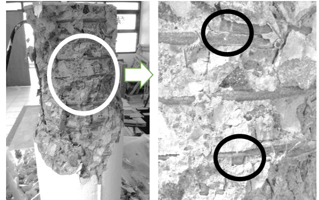
Gambar 14. Detail kegagalan tulangan pengekan tidak standar
