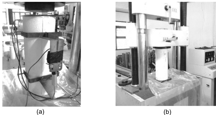
Gambar 6. Setup alat pengujian (a) Posisi LVDT pada benda uji (b) Benda uji pada UTM
