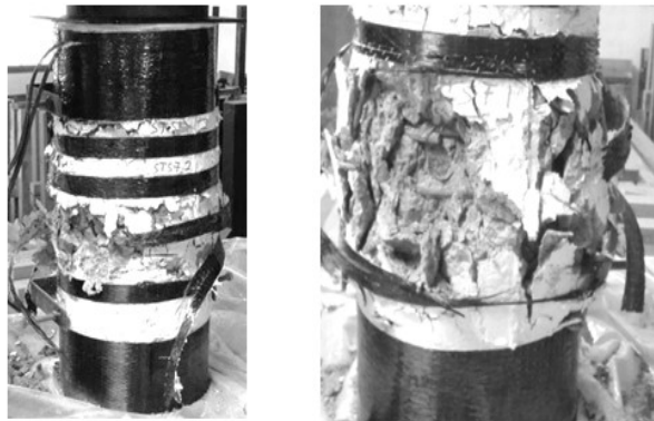
Gambar 12. Detail kegagalan tulangan pengekan tidak standar dengan perkuatan FRP
