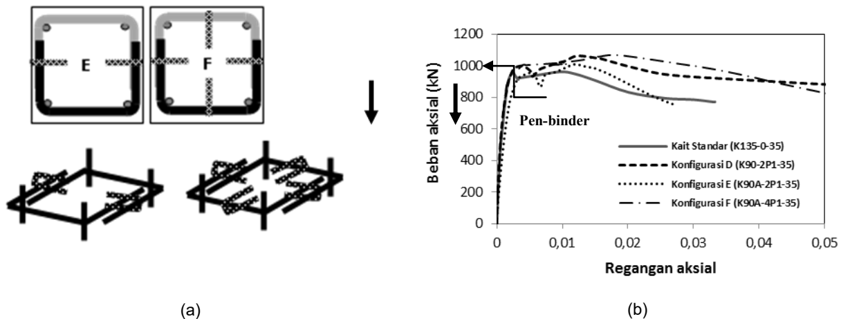
Gambar 1. (a) Konfigurasi pemasangan pen-binder pada kolom persegi (b) Hasil pengujian penggunaan pen-binder sebagai perkuatan tulangan pengekan pada kolom persegi (Kristianto, dkk., 2012)
