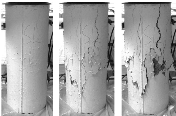
Gambar 13. Pola retak benda uji kolom lingkaran tulangan pengekan tidak standar
