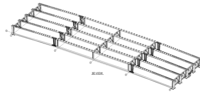
Gambar 4. Struktur jembatan girder
