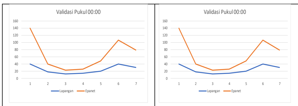
Gambar 5 Hasil validasi tekanan model epanet
